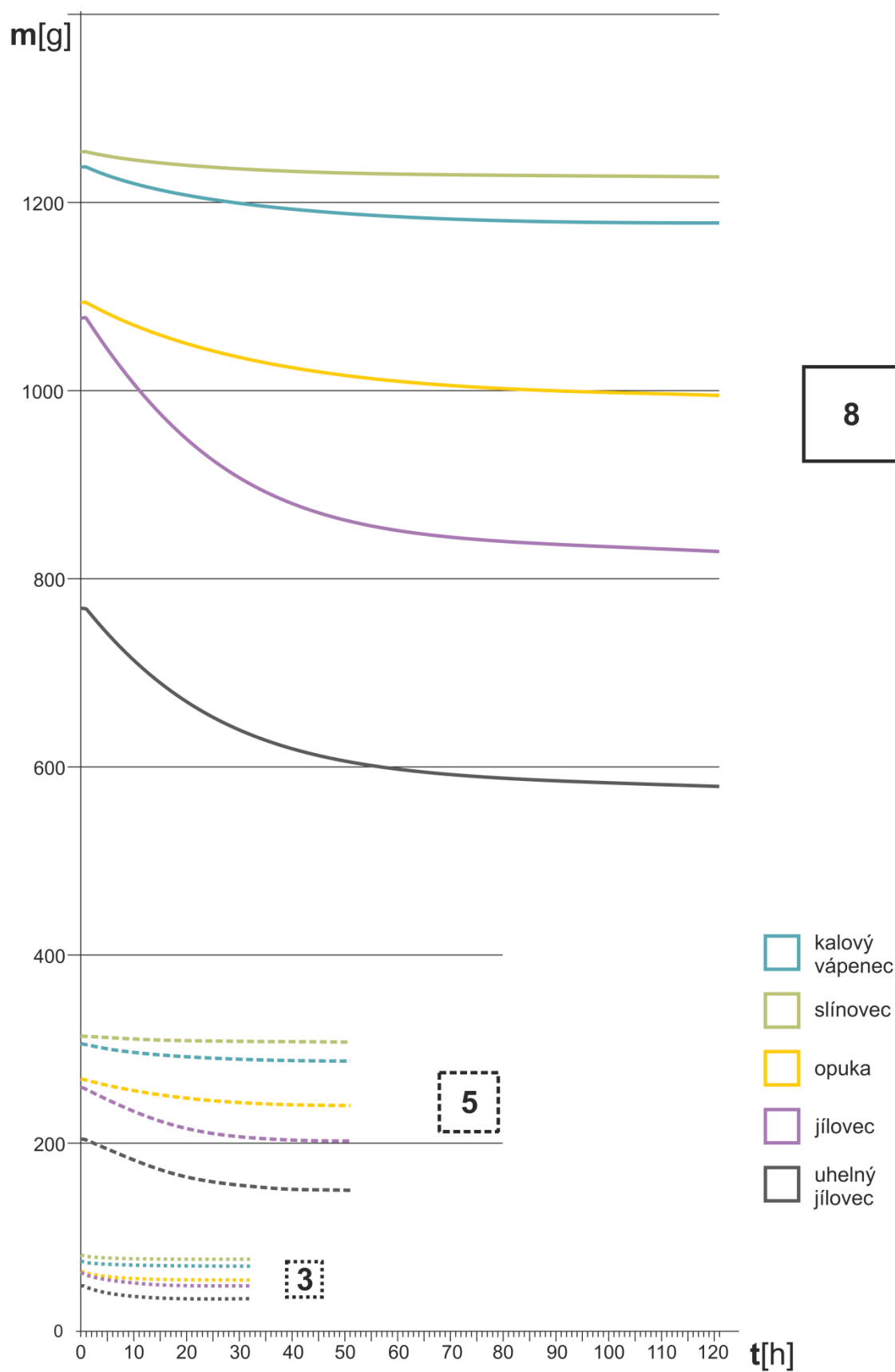
Obr. 10-1 Diagram srovnávající rychlosti vysoušení vybraných hornin lyofilizací – vyjádřeno ztrátou hmotnosti za jednotku času
